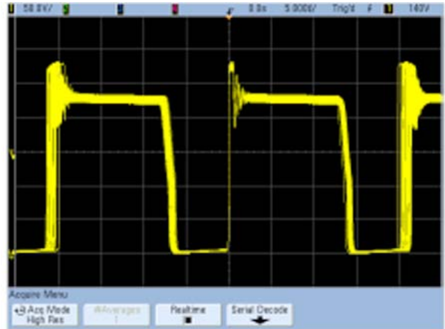
Рис. 3. Сигнал напряжения V_{ds} импульсного источника питания, захваченный в режиме высокого разрешения.
